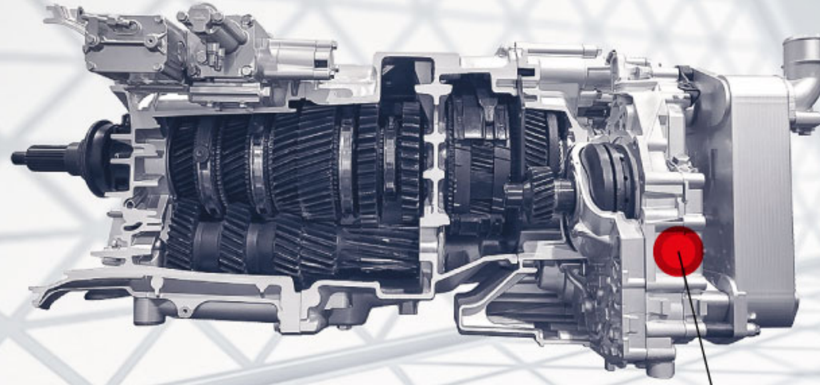
ناقل الحركة يدوي بـ 5 سرعات 5-Manual Transmission
